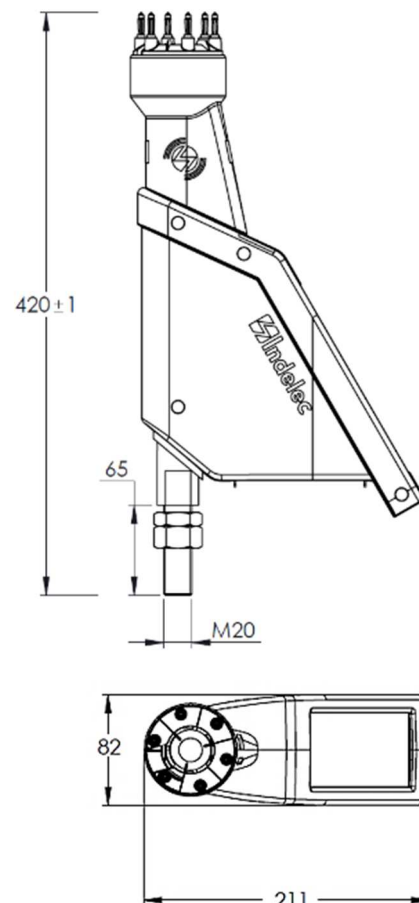
Rozměry (mm)
